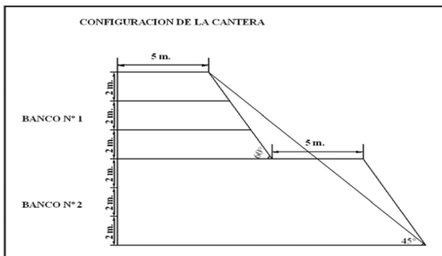
Figura N° 3.2: Dimensiones del banco, berma y talud
